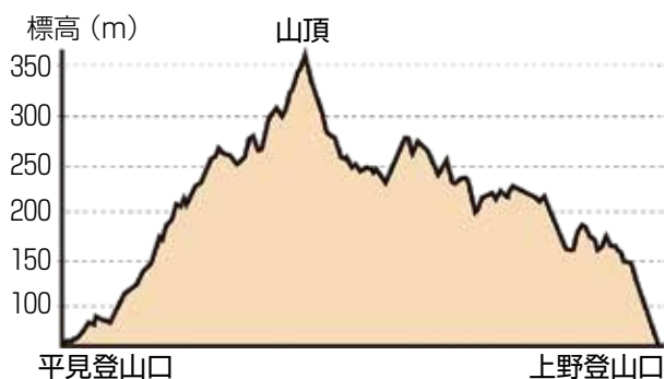
図. 大烏帽子山（平見～上野登山口）断面図
