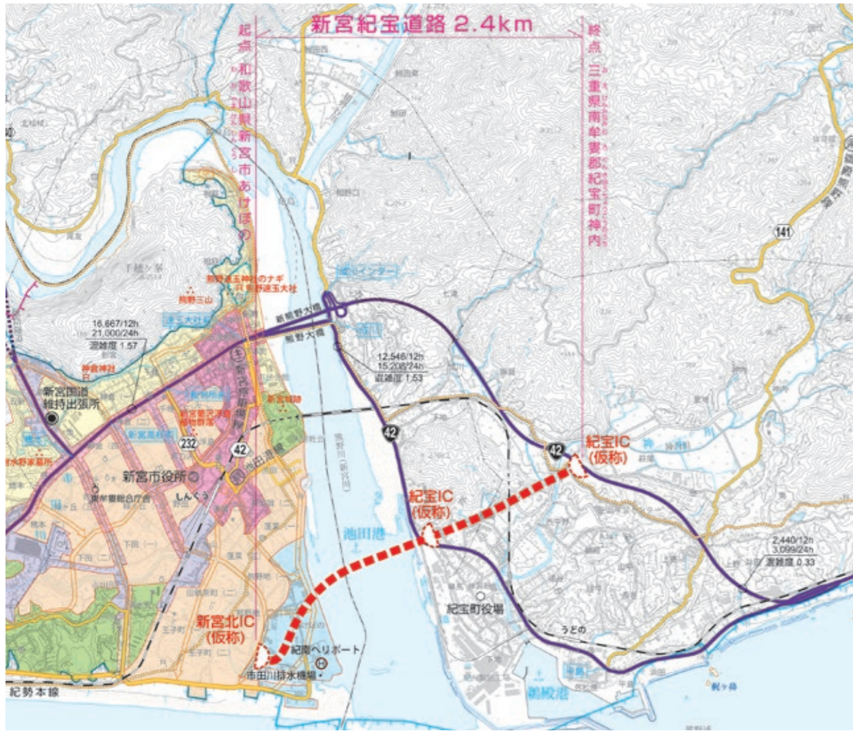
新宮紀宝道路の計画位置図
