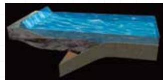
④ 津波が沿岸部に到達する
