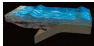
③ 津波が海面を伝わり四方八方に広がる
