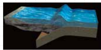
② 地殻変動に合わせて海面が持ち上げられる
